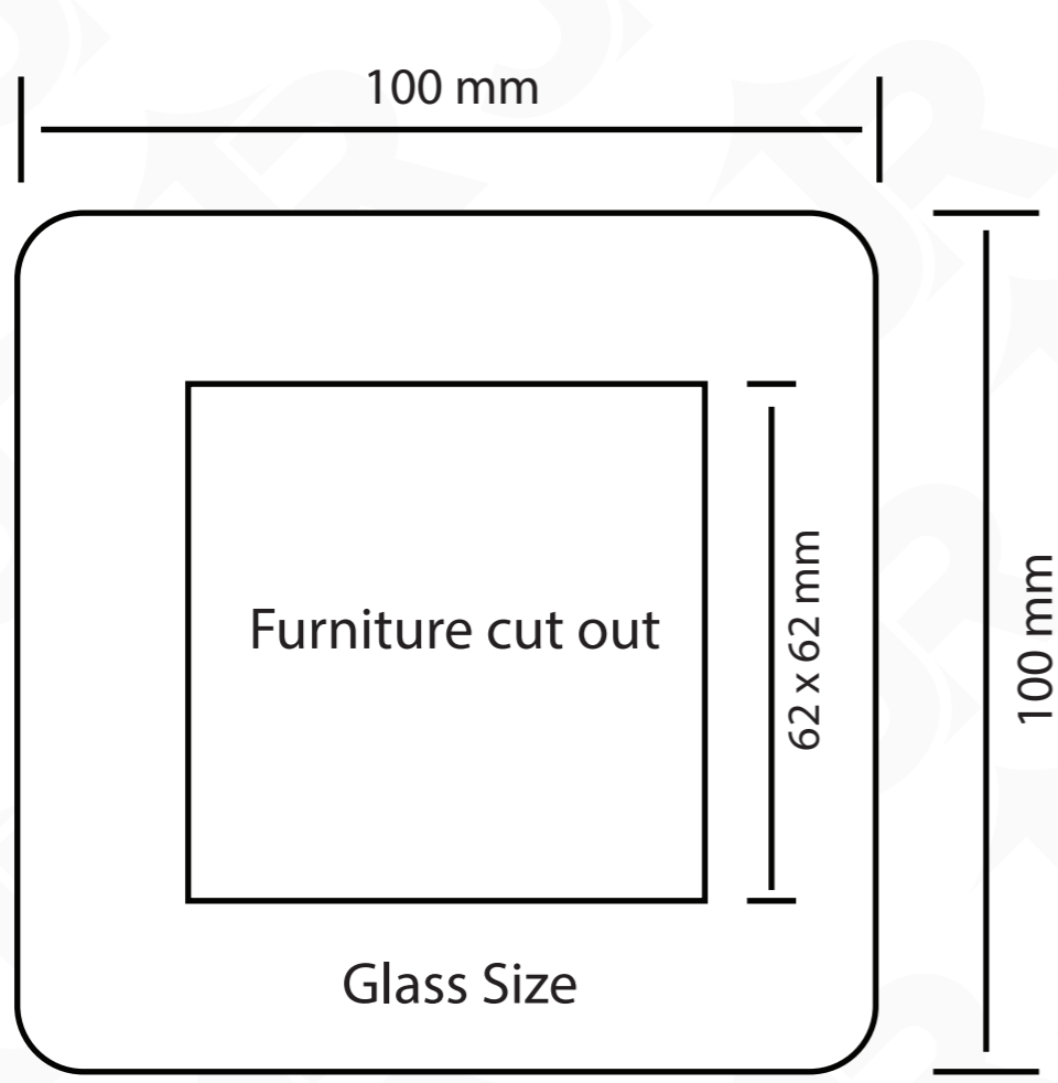
2 Module
