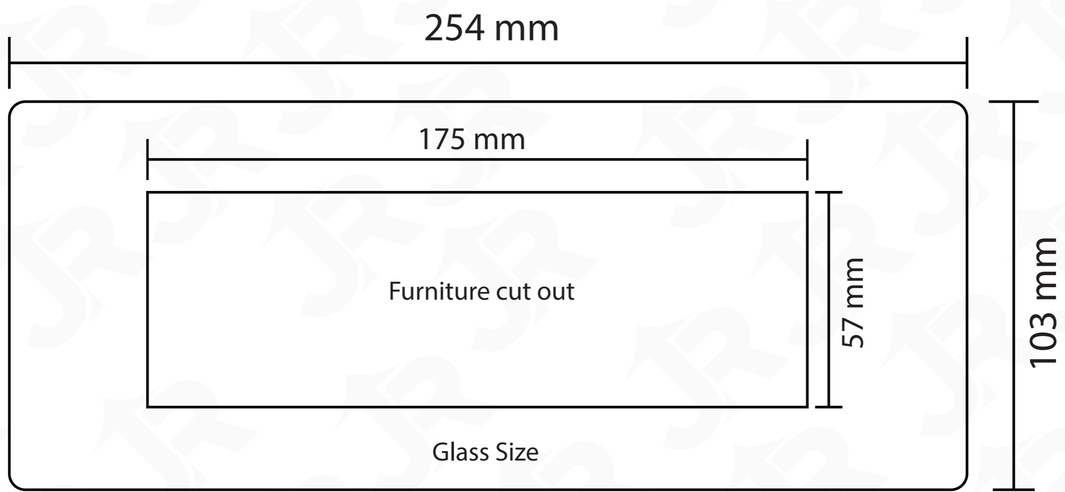
6 & 8 Module
